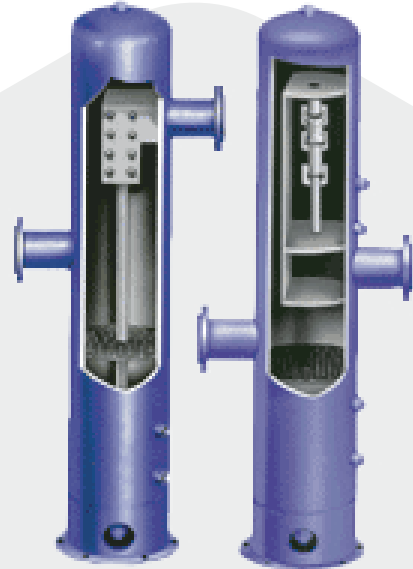
Scrubbers y Separadores Tipo Ciclótubo y Tipo Vena 3 - 10 \mu m
