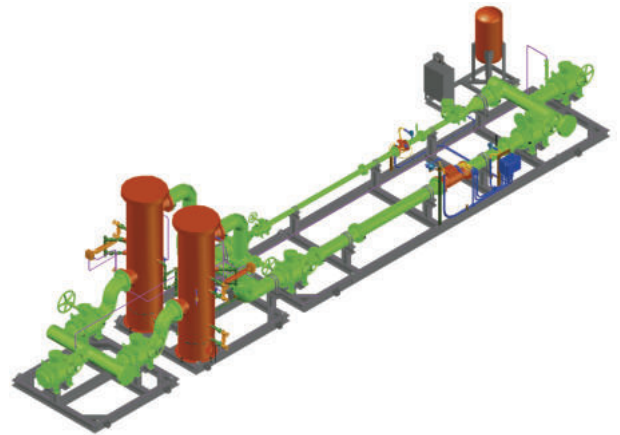
Ingeniería de Detalle Skid de Medición y Odorización EMO-PILAT
