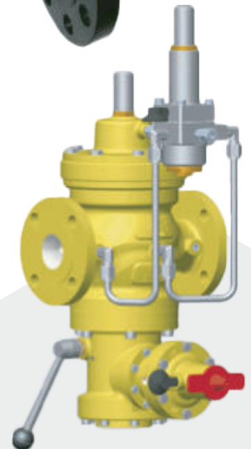
Válvula Reguladora de Presión con Shut-Of Incorporada ARGOS + SSV
