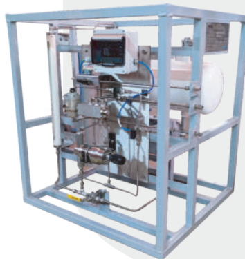
Odorizador de micro caudales X1 - Portatil
