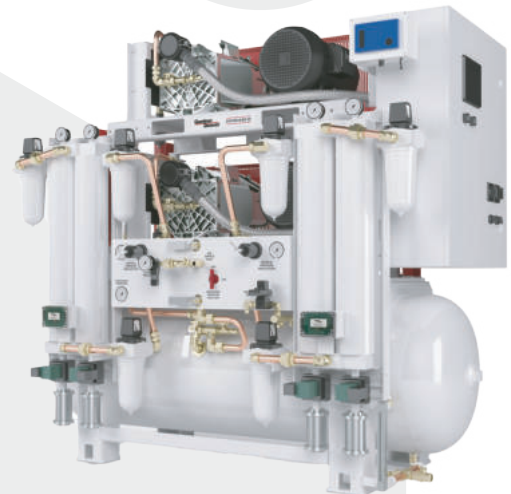
Estación de Compresión de Aire Medicinal NFPA 99 Tipo Scroll con Monitor de CO2 y Tanque Pulmón
